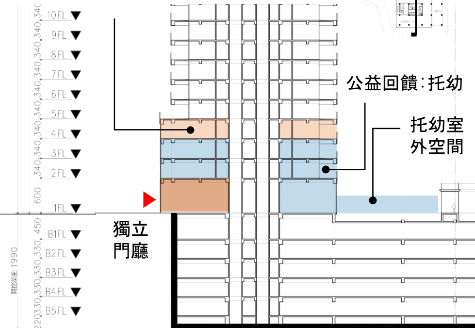
特專三 E棟 示意剖面
